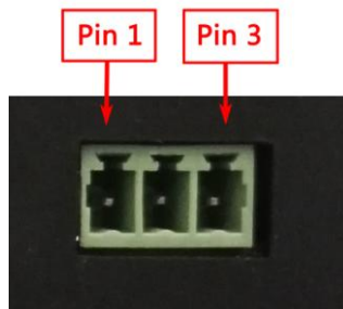
图片3 电源输入接口
